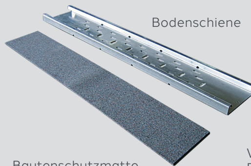
Bautenschutzmatte (Stärke mindestens 4–8 mm)
