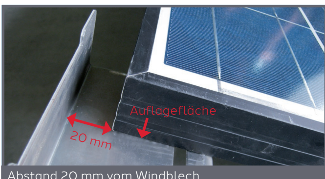
Abstand 20 mm vom Windblech
