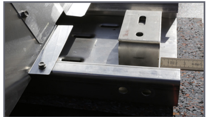
Abstand von min. 20 mm zum Bodenschienen-Ende
