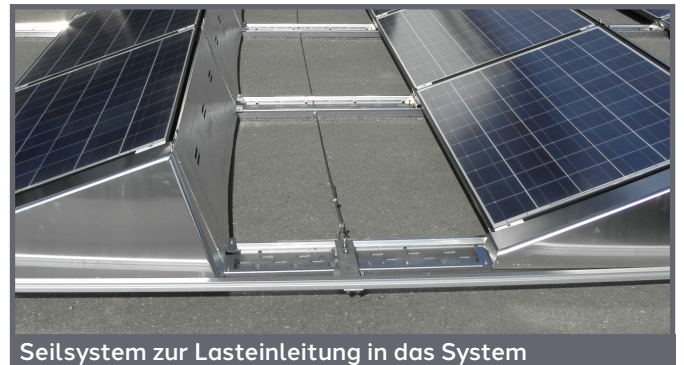
Seilsystem zur Lasteinleitung in das System
