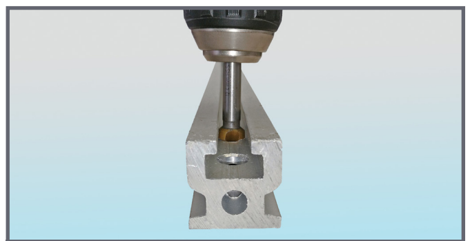
... Löcher innen senken mit Spezialsenker
