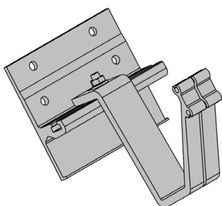
Dachhaken variabel Für Falzziegel & Betonziegel, seitlicher Verstellbereich 100 mm.
