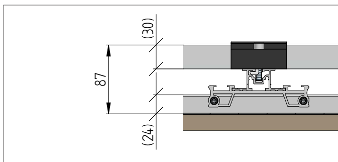
Duramont Klemmsystem light für Blechfalzdächer
