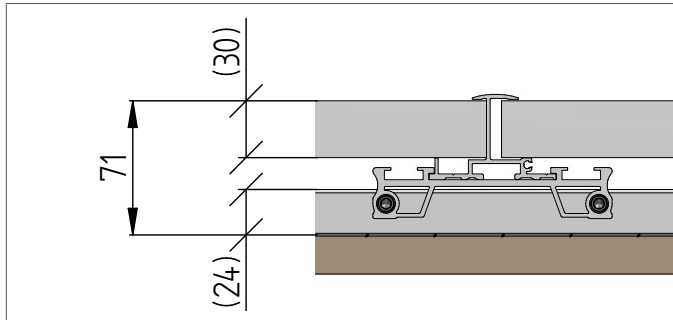
Duramont Einlegesystem für Blechfalzdächer
